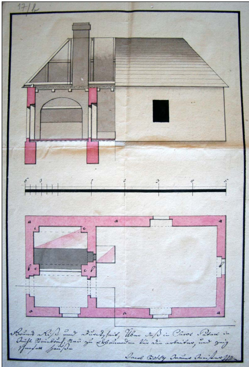
5. kép. A malomkőbánya műhelyének terve, 1802 (SRKTGY Kt 1625/17/b) (Fotó: Marozsán Zsolt) Fig. 5. Plan of the manufactory of the millstone-quarry, 1802 (Scientific Collection of the Calvinistic College of Sárospatak, Kt. 1625/17/b) (Photo by Zsolt Marozsán)
