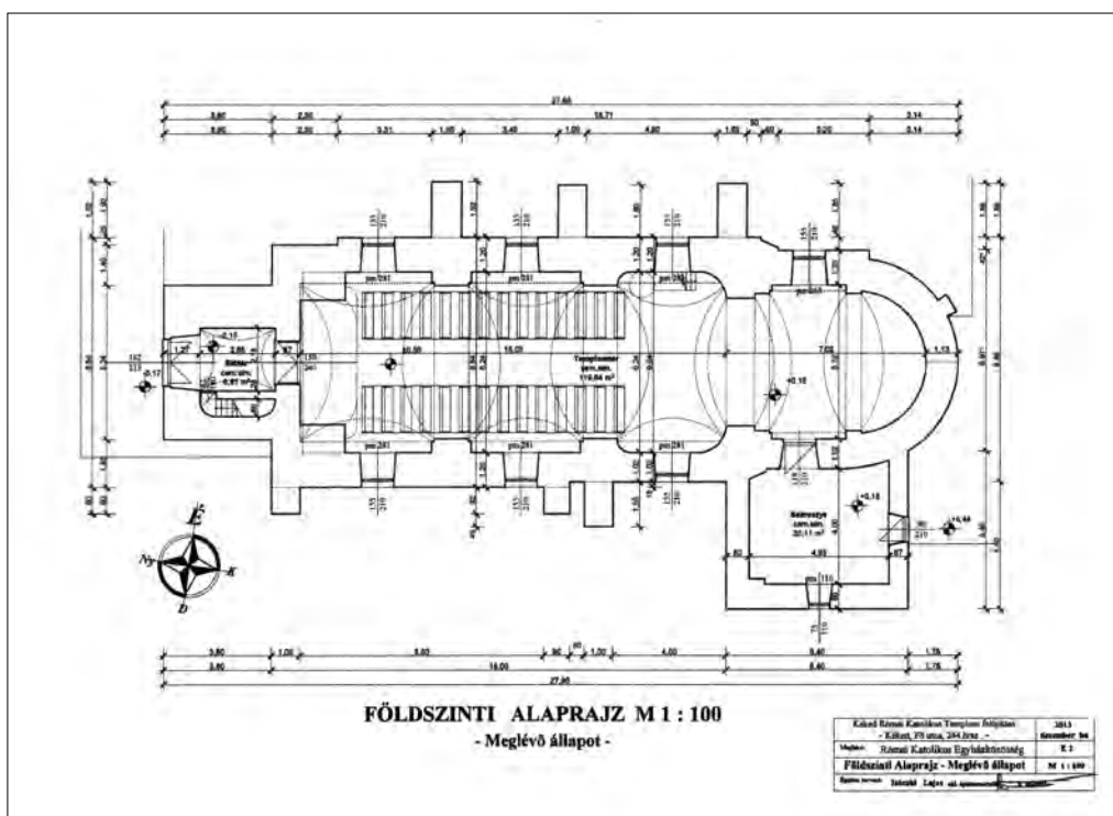
3. kép A templom alaprajzi felmérése, 2013. Isóczki Lajos okl. építészmérnök munkája.
